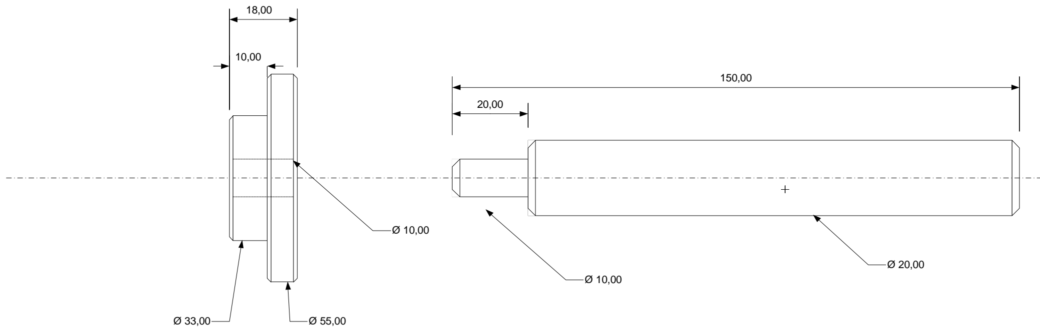
outil de mise en place du joint SPI
